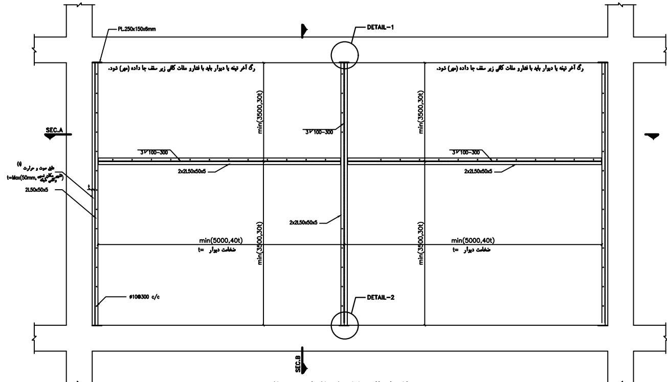
جزئیات اجرایی دیوارهای غیرسازه ای بدون بازو Sc. 1:25
