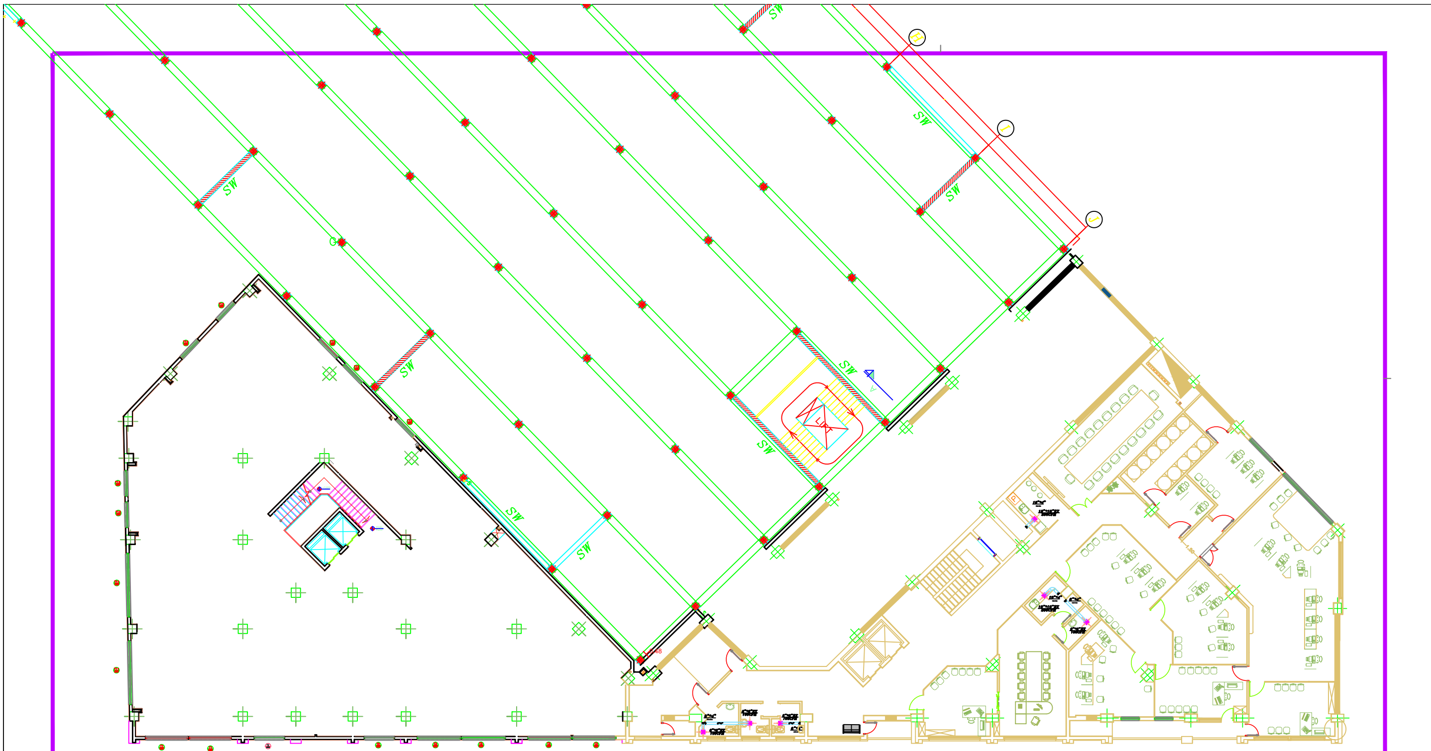
پلان طبقه اول
