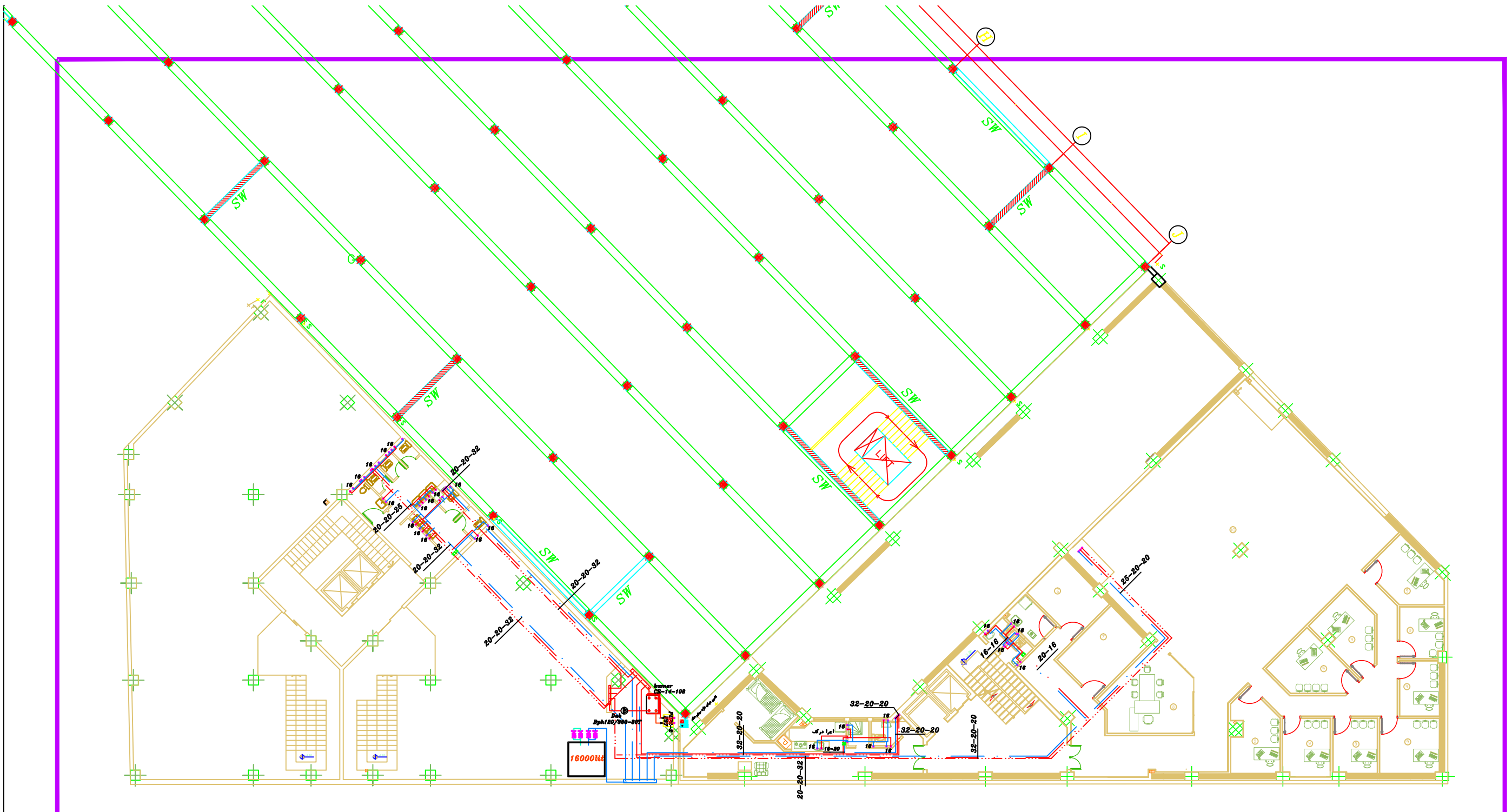
پلان طبقه زیرزمین ۲-
