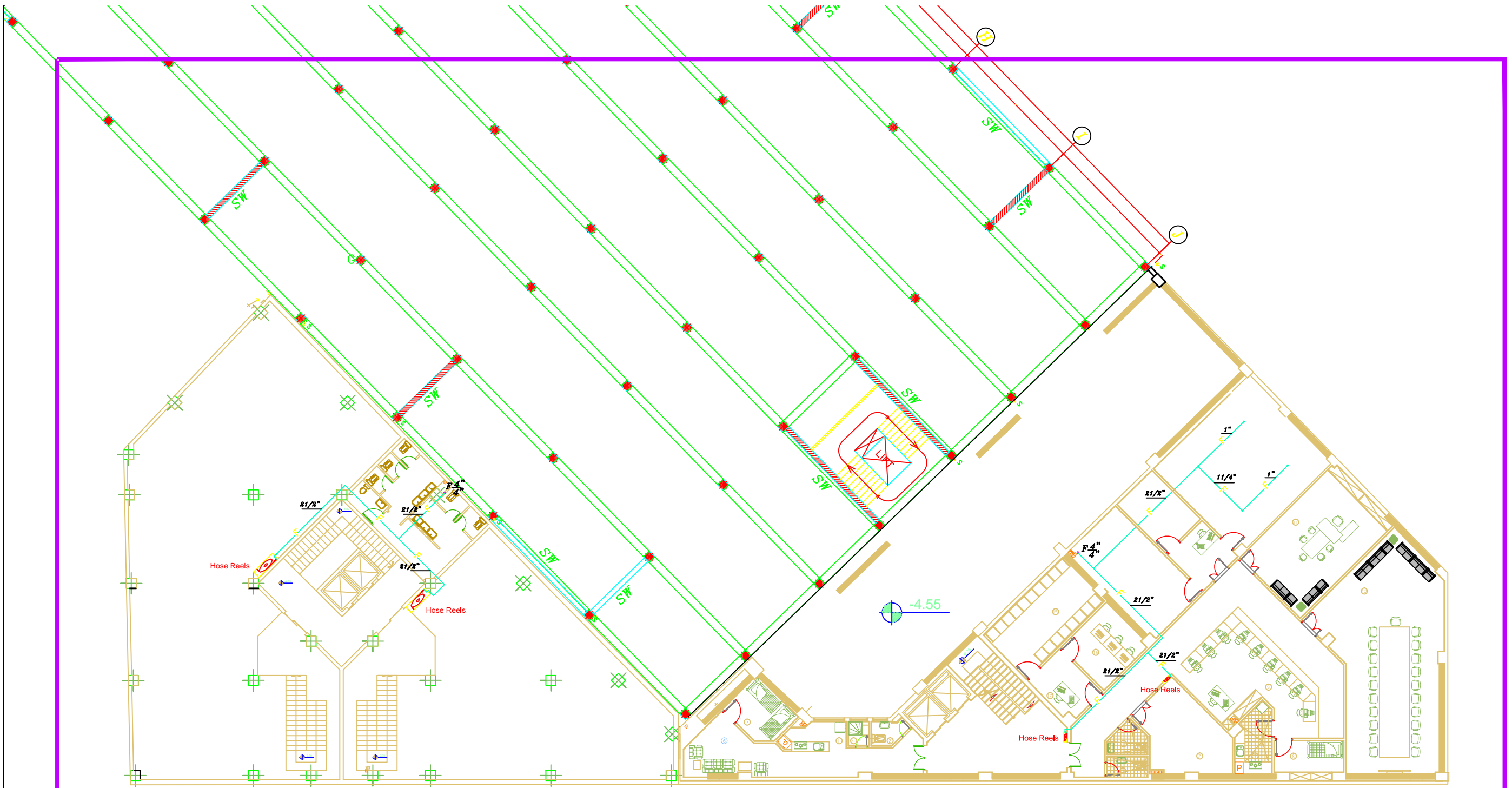
پلان طبقه زیر زمین ۱-
