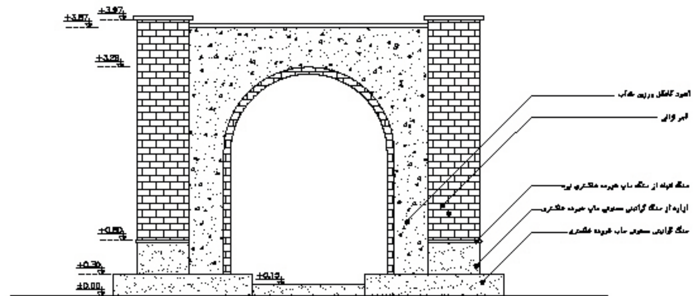
جزئیات نمای طاق EL-03 A3-16
