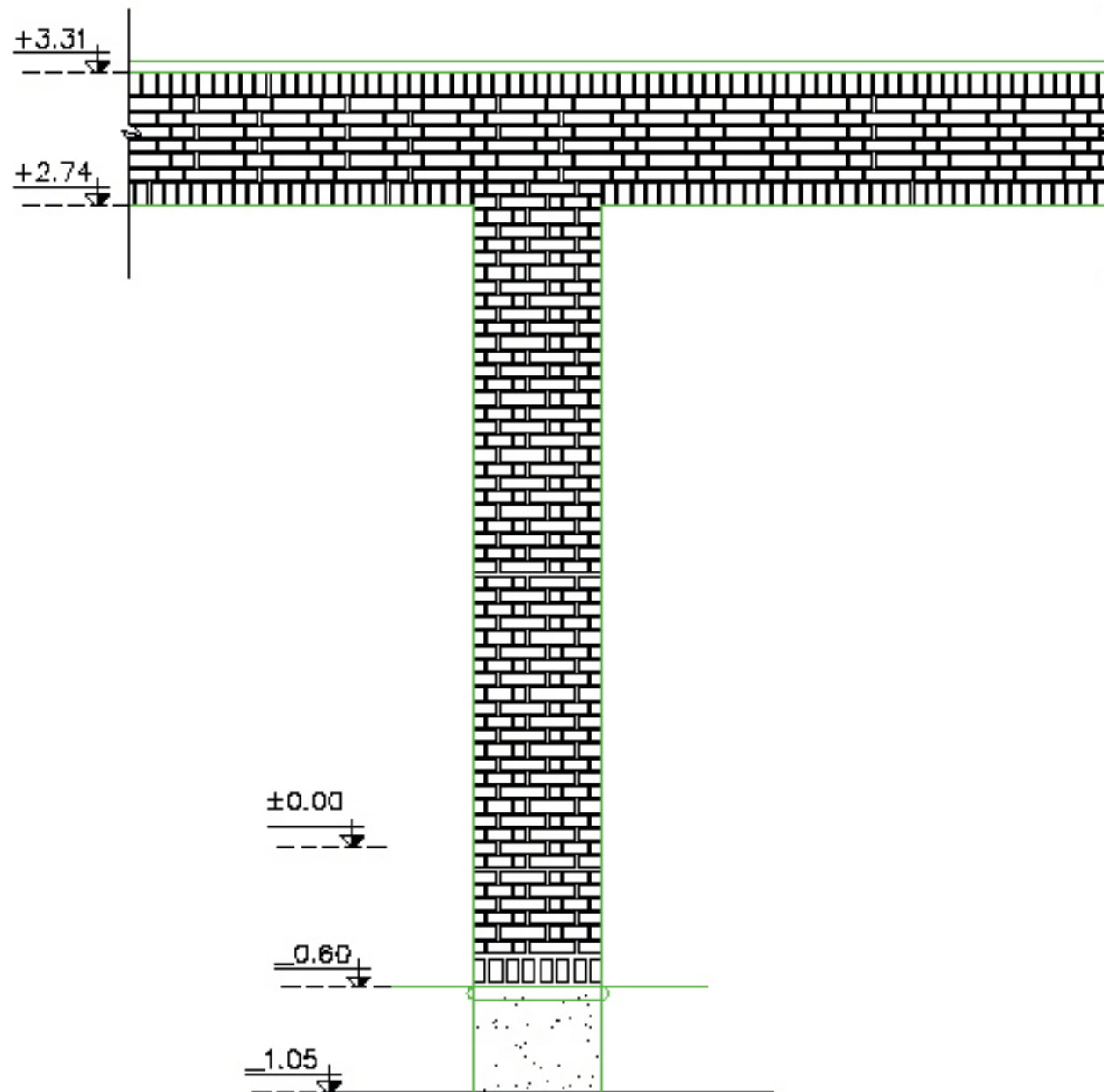
جرمیات آجرکاری نما 1a-1b A3-B3
