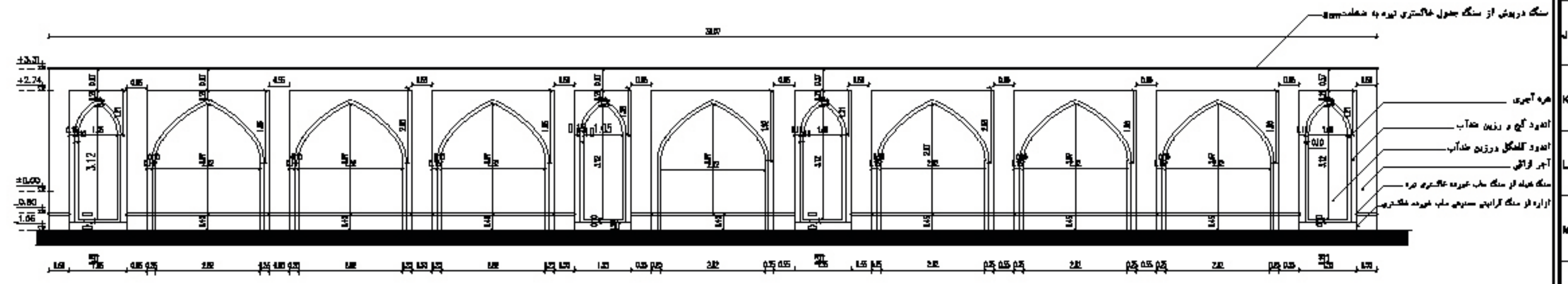
اندازه گذاری نما EL-08 AS-26
