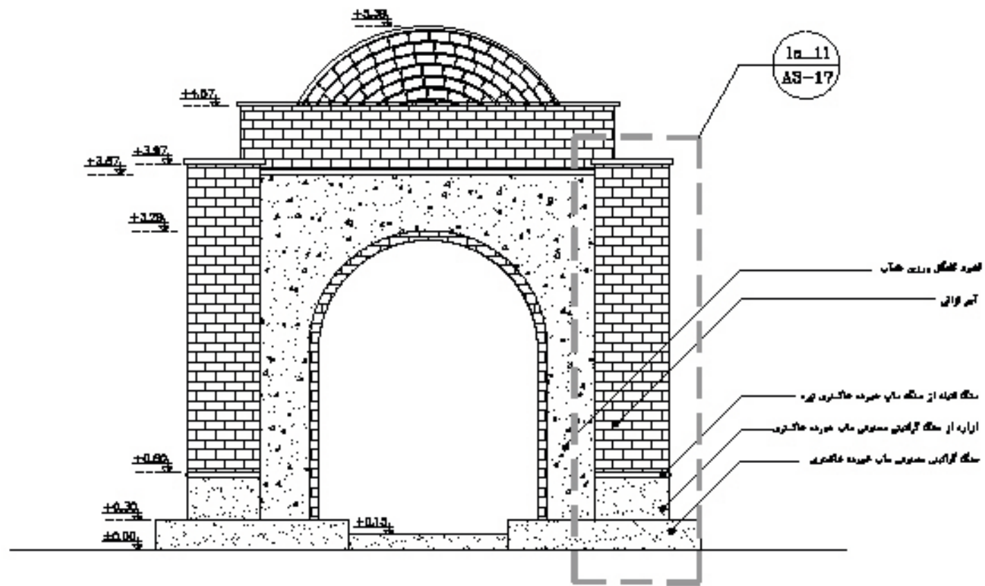
جزئیات نمای طاق: 04-04 AS-14
