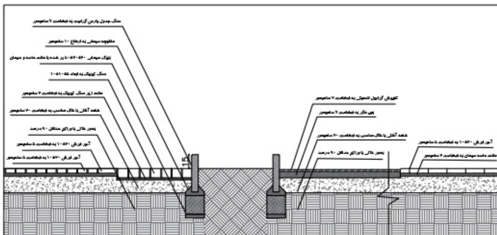
SEC : C-C
