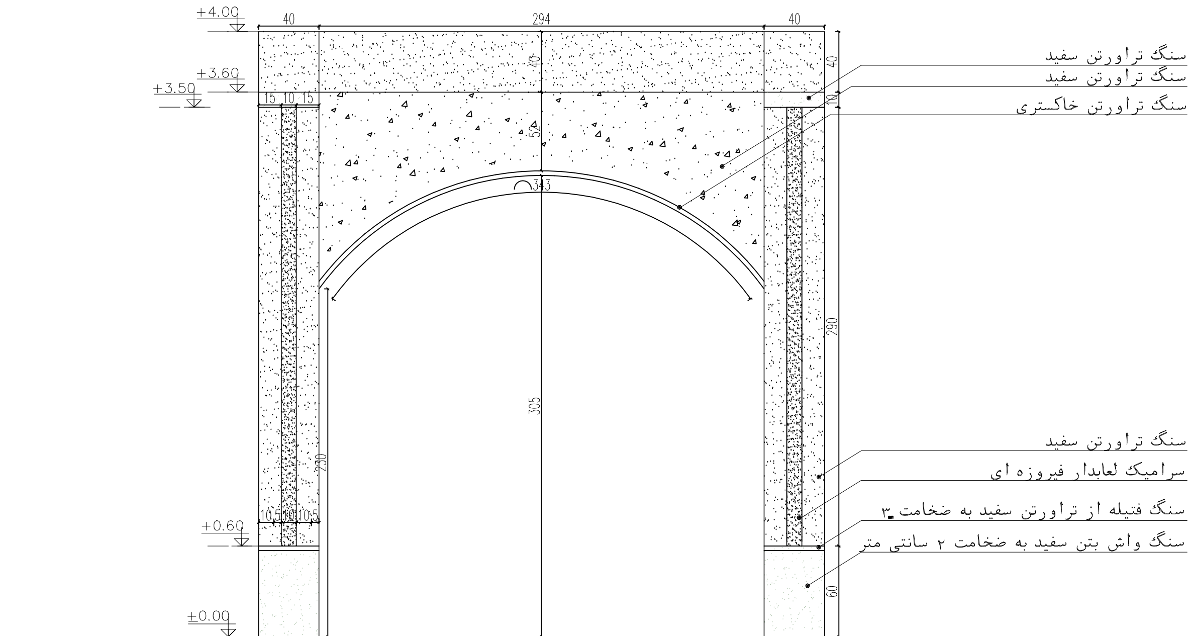
جزئیات نمای طاق EL-1 A3-07 sc-1.25
