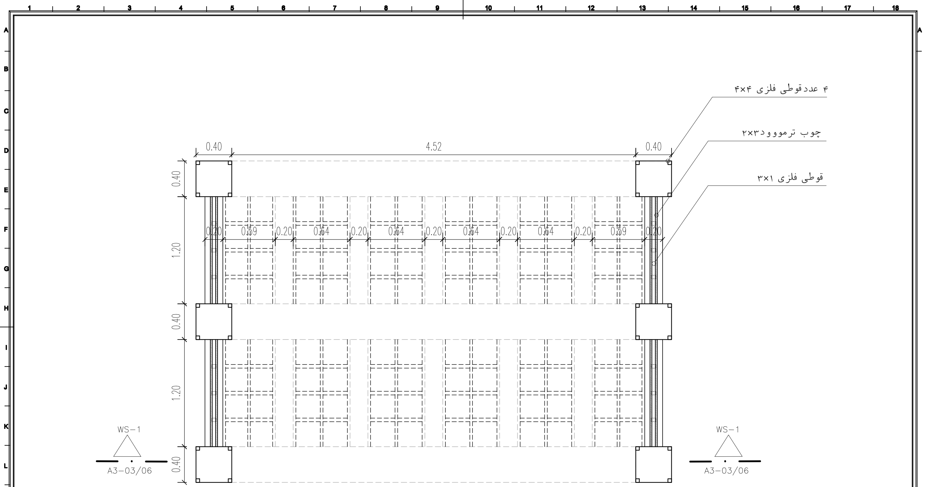
جزئیات ورودی اصلی from at elevation +1.02 det02
