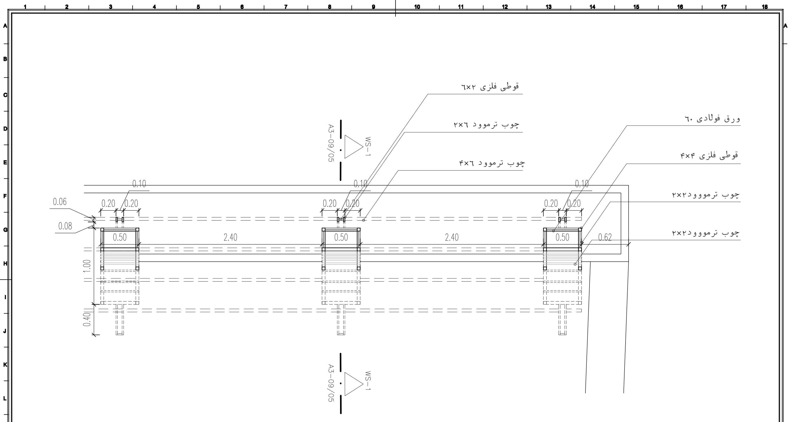
جزئیات مسیر منتهی به پارک بانوان LA-04 A3-09 from at elevation +1.00
