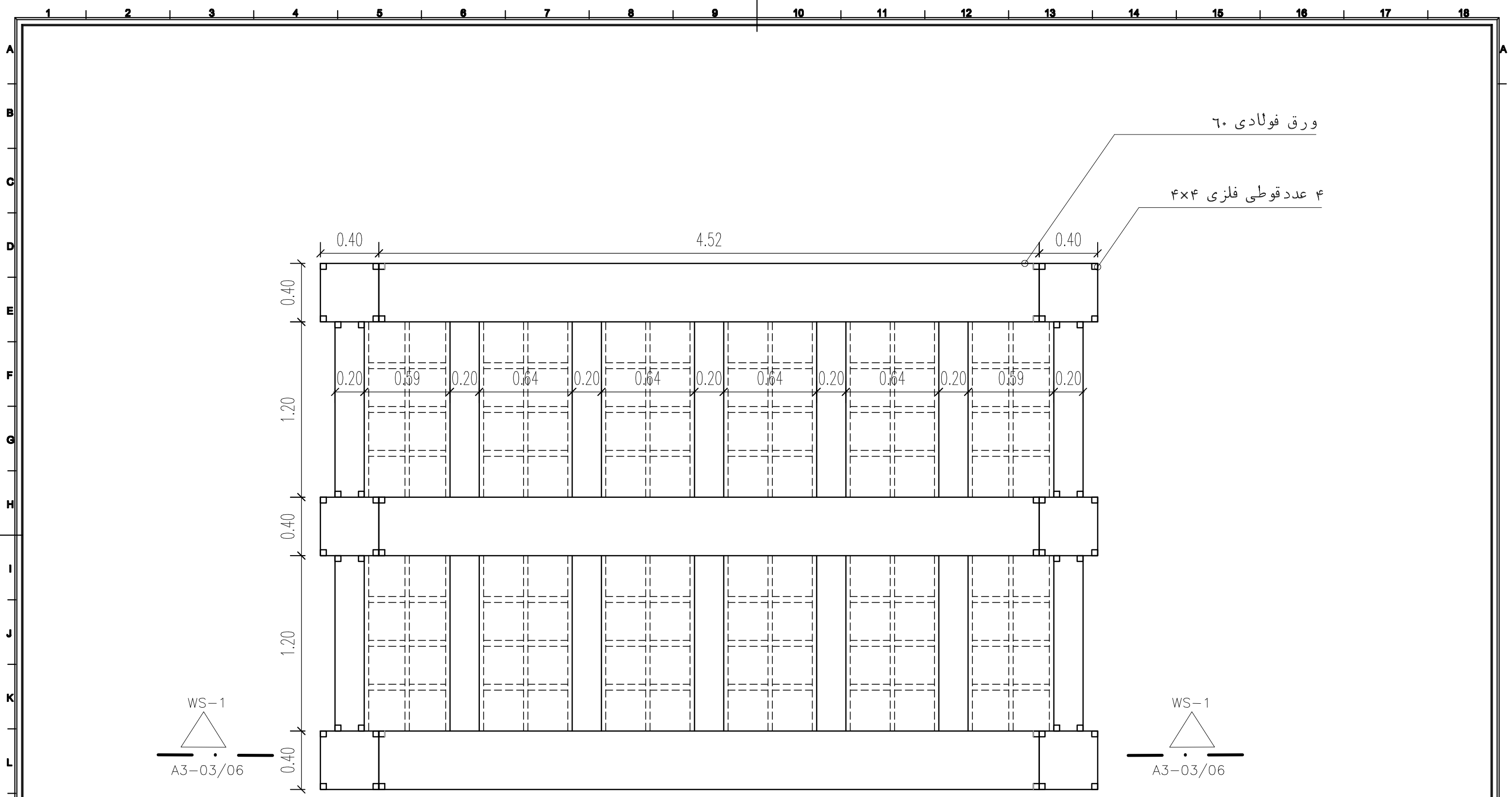
جزئیات ورودی اصلی det02 from at elevation +2.90
