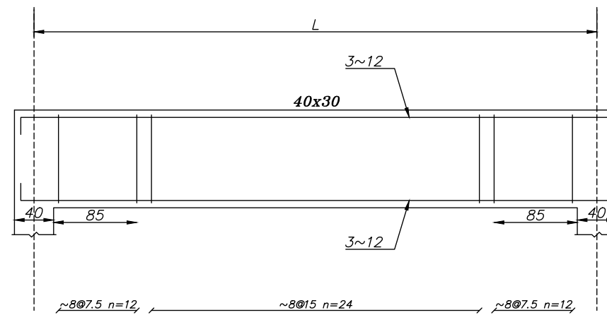
Beam Typ. B
