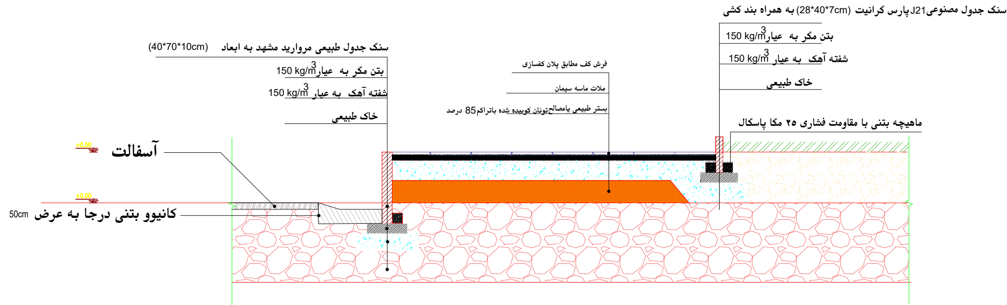
جزئیات اجرایی مقیاس : 1/100 detA-A
